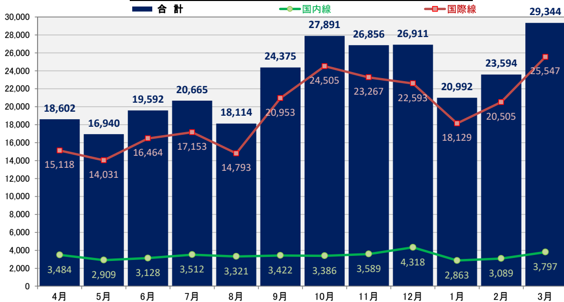
[iii] 中部国際空港 2005年度月次別 貨物取扱量(単位:トン)
