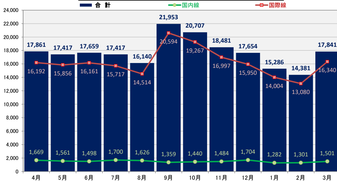
[iii] 中部国際空港 2018年度月次別 貨物取扱量(単位:トン)
