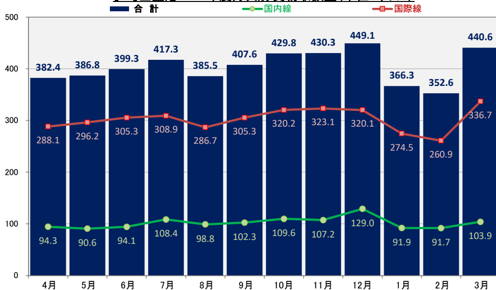
[iii] 全空港 2024年度月次別 貨物取扱量(単位:千トン)
