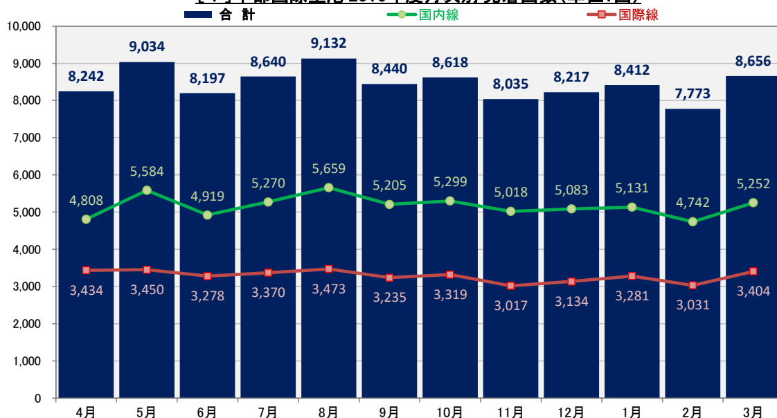
[i] 中部国際空港 2016年度月次別 発着回数(単位:回)
