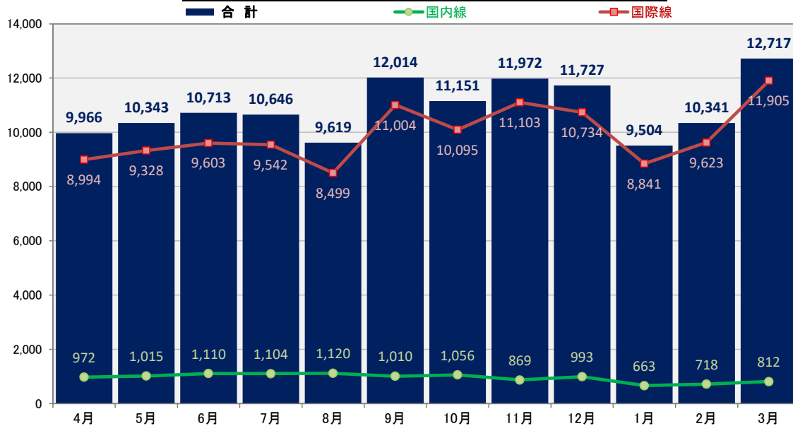
[iii] 中部国際空港 2023年度月次別 貨物取扱量(単位:トン)
