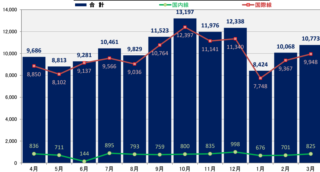
[iii] 中部国際空港 2022年度月次別 貨物取扱量(単位:トン)
