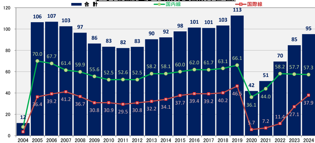
[i] 中部国際空港 年度別 発着回数(単位:回)
