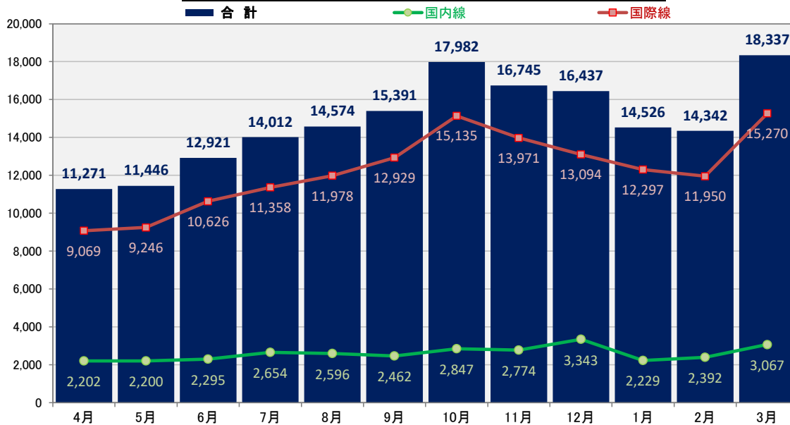
[iii] 中部国際空港 2013年度月次別 貨物取扱量(単位:トン)
