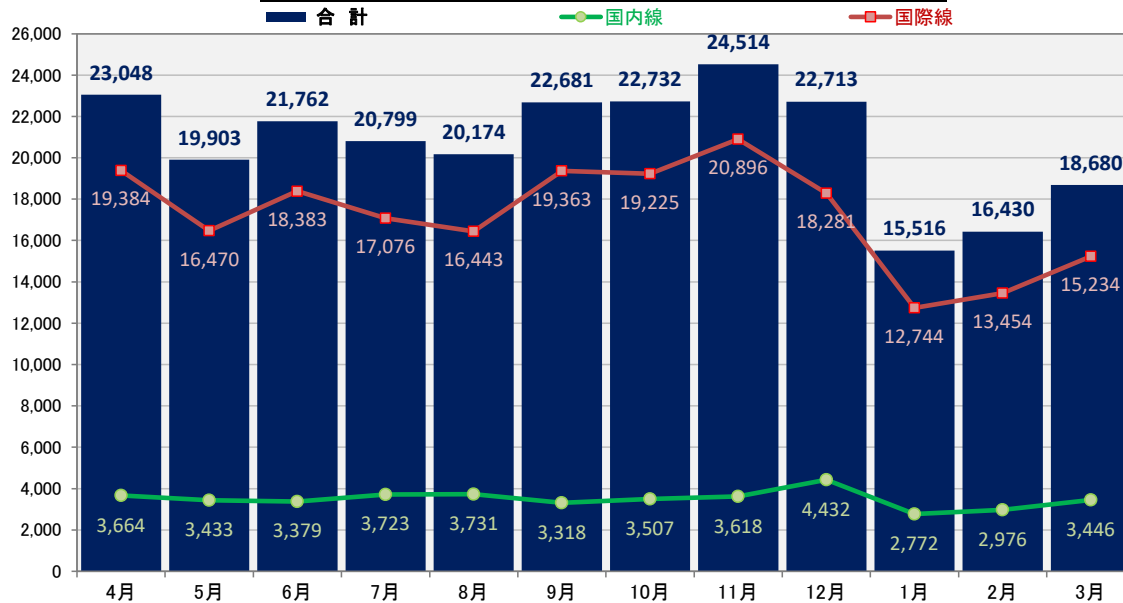
[iii] 中部国際空港 2007年度月次別 貨物取扱量(単位:トン)
