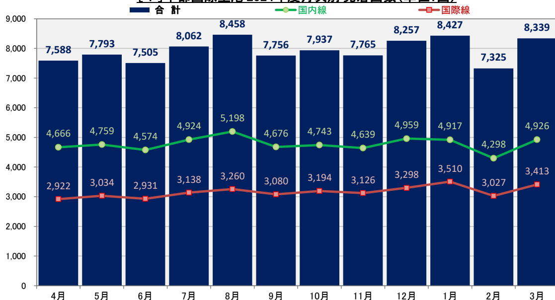
[i] 中部国際空港 2024年度月次別 発着回数(単位:回)
