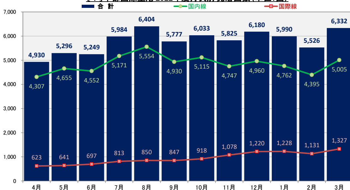
[i] 中部国際空港 2022年度月次別 発着回数(単位:回)
