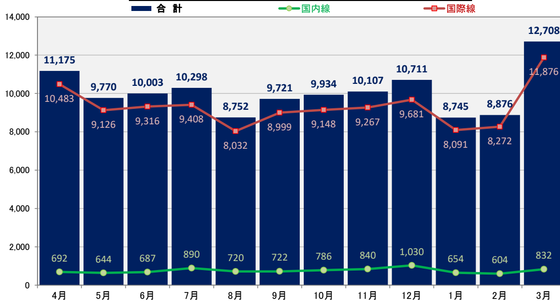
[iii] 中部国際空港 2021年度月次別 貨物取扱量(単位:トン)
