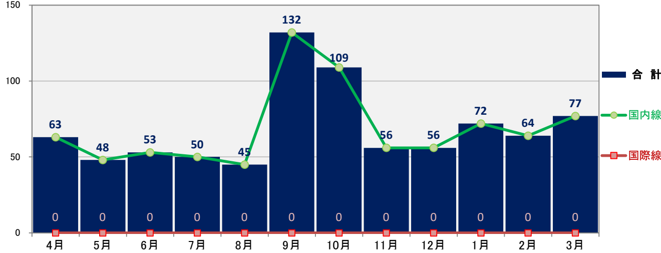
[iii] 能登空港 2024年度 月次別 着陸回数(単位:回)
