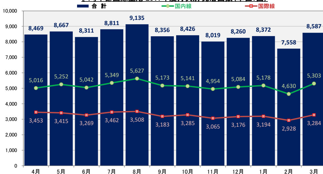
[i] 中部国際空港 2017年度月次別 発着回数(単位:回)
